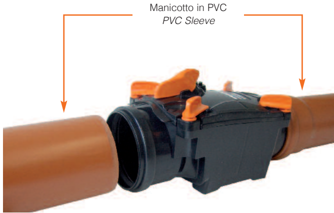
Esempio di installazione su tubazioni in PVC o PP. Example of installation on existing pvc or pp pipes.
